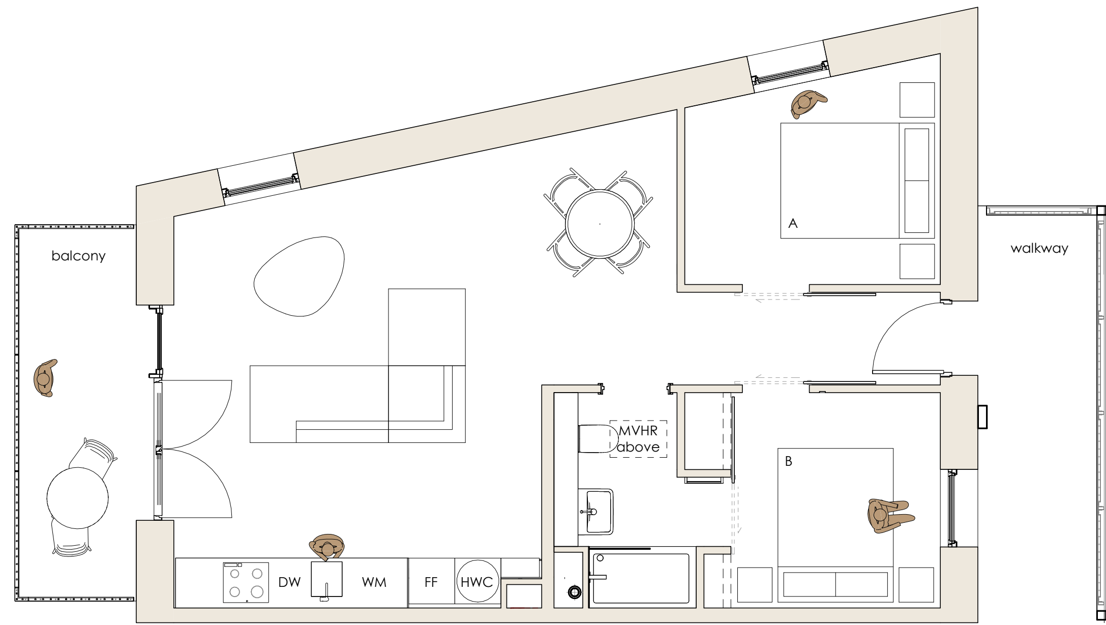
PLAN 1:50
